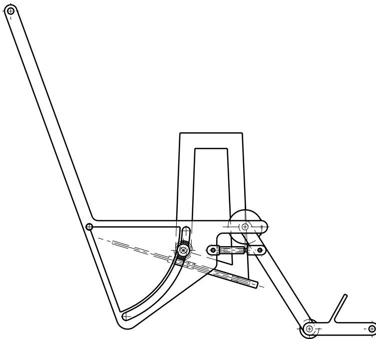
Vista frontal Escala: 1:12
